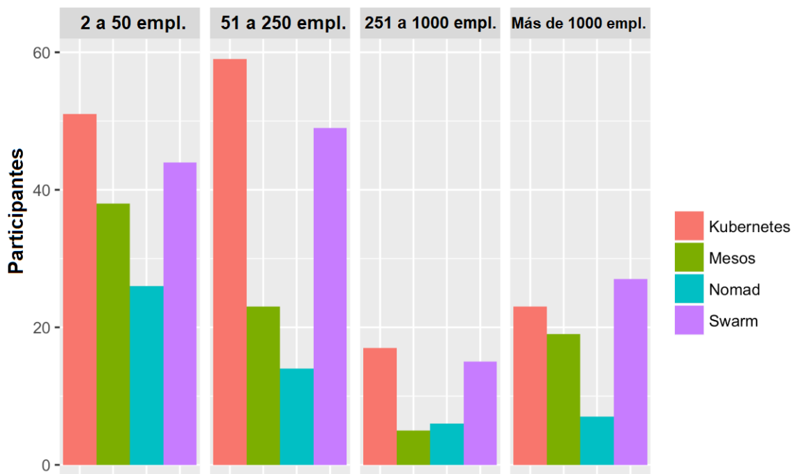
Figura 3.3: Orquestadores utilizados por compañías según su tamaño (en número de empleados).
