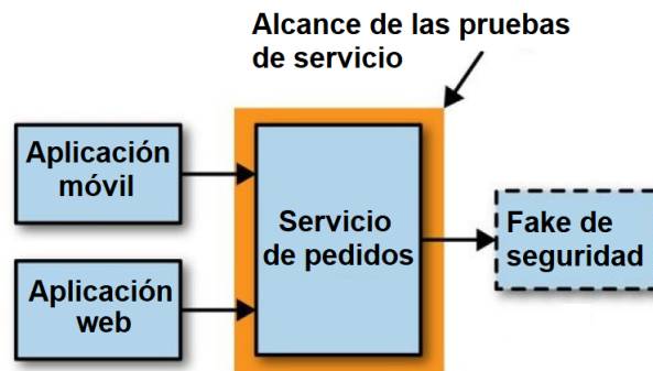
Figura 2.8: Diagrama de pruebas de servicios.
