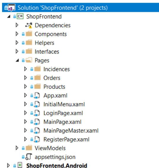
Figura 6.19: Solución de la interfaz de usuario hecha con Xamarin.Forms.
