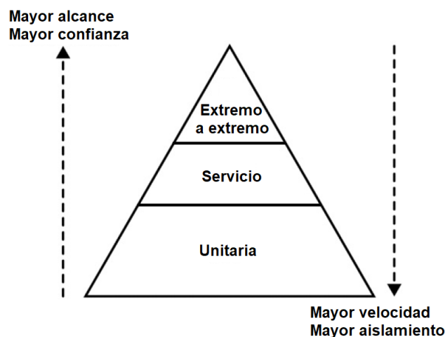
Figura 2.10: Pirámide de pruebas diseñada por Mike Cohn [8].
