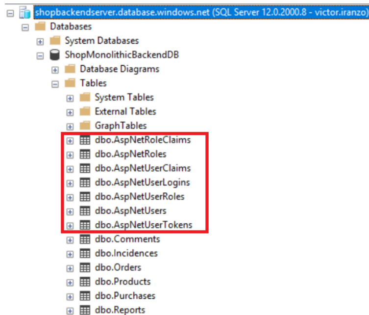
Figura 6.6: Tablas creadas por ASP.NET Core Identity.
