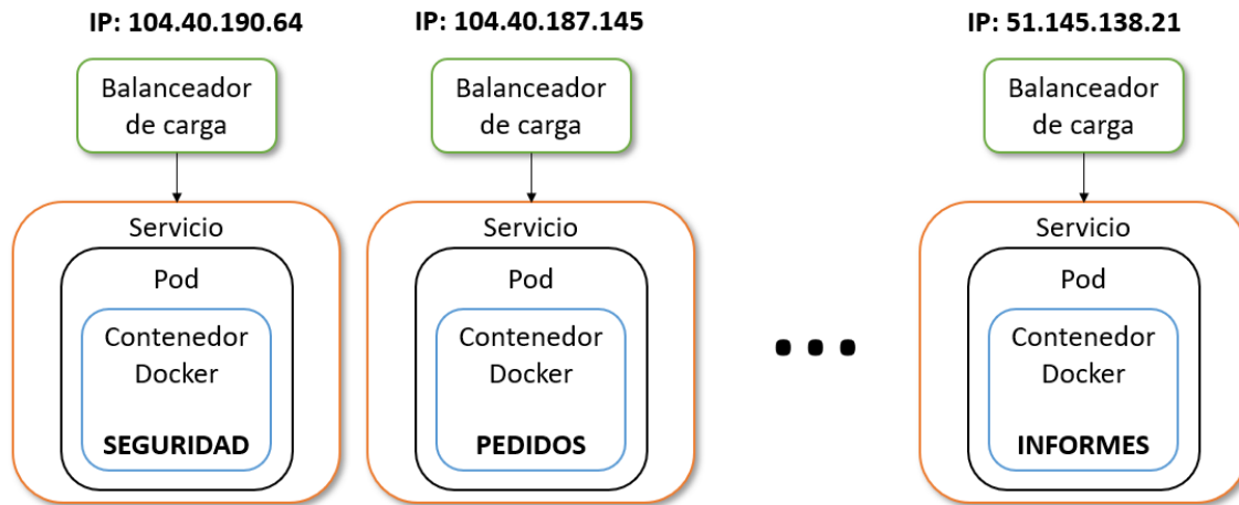
Figura C.12: Representación del despliegue en producción.
