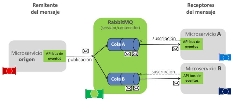
Figura 2.5: Ejemplo de integración basada en eventos con un contenedor de RabbitMQ [12].
