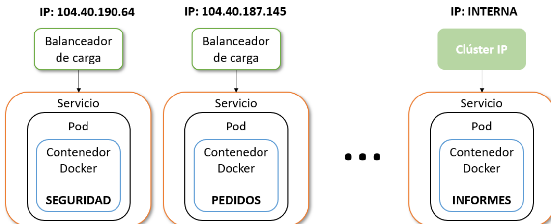
Figura C.13: Uso de ClusterIP en el microservicio de informes.
