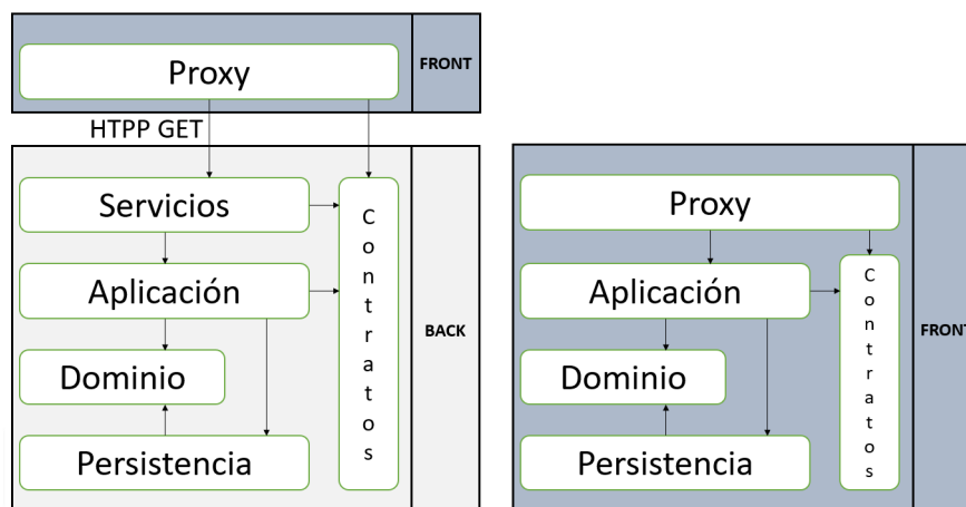
Figura 6.18: Sistema de back-end como un servicio (izquierda) y como una librería (derecha).
