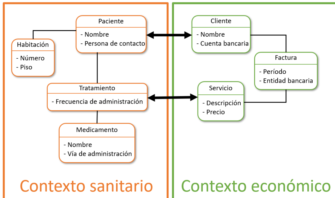
Figura 2.3: Ejemplo de dos contextos delimitados.
