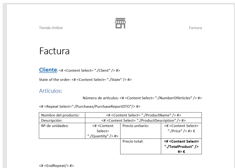
Figura 6.13: Plantilla para la creación de facturas.
