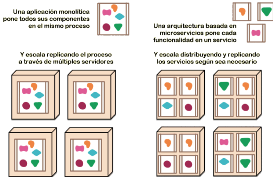
Figura 2.1: Escalabilidad en los microservicios [25].
