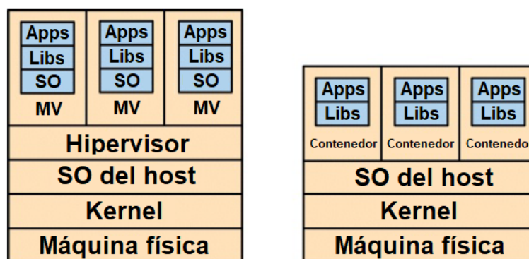
Figura 2.12: Comparación entre la virtualización (izquierda) y la contenerización (derecha) [33].
