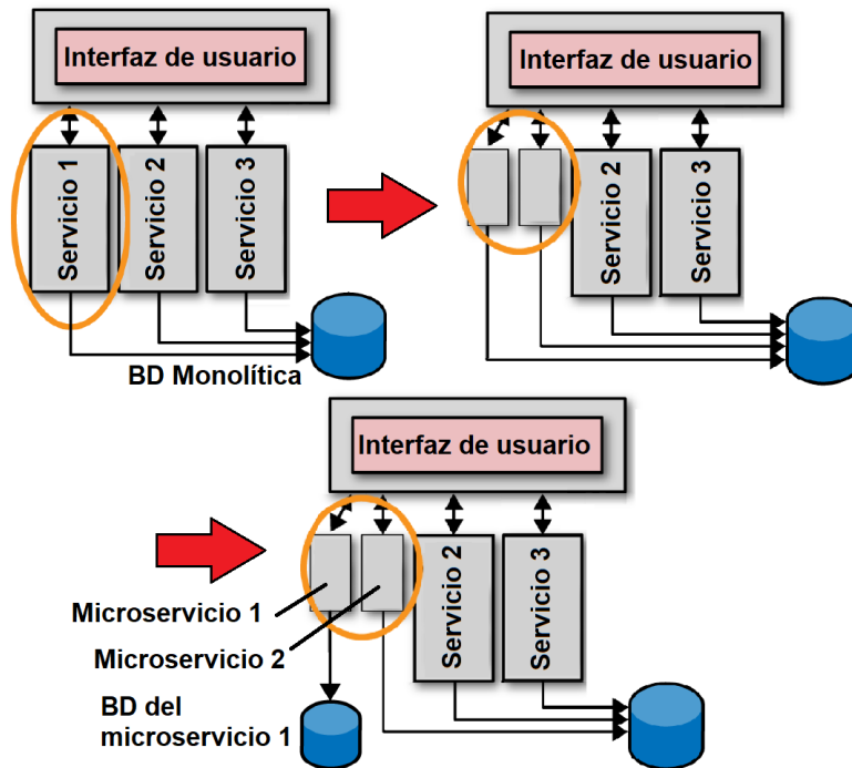
Figura 2.4: Descomposición de un servicio en dos [38].
