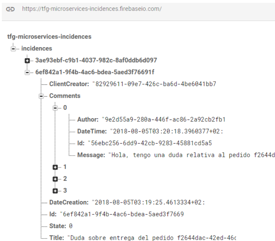
Figura 7.9: Base de datos de incidencias en Firebase.
