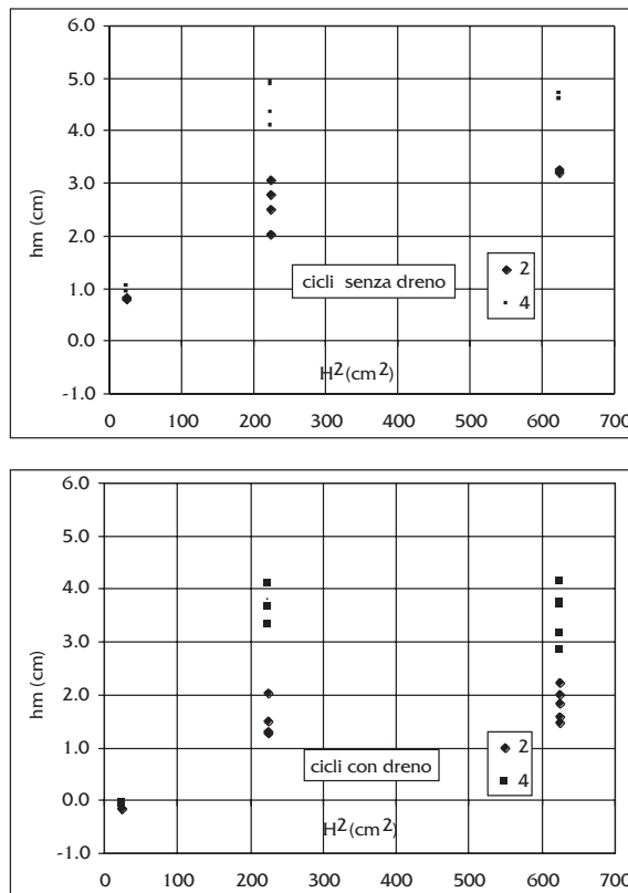
Figura 12. Andamento della quota massima della W.T. (trasduttore 4) e di quella in corrispondenza del dreno (trasduttore 2) in funzione di H²
