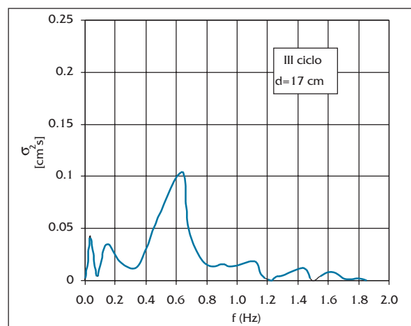
Figura 4. Spettro di ampiezza dell'altezza d'onda al largo (d=80cm) e sottocosta (d=17cm)
