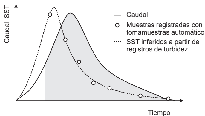
Figura 5. Esquema típico de registro de la contaminación con un tomamuestras automático con alarma de inicio tras superar cierto umbral de caudal o nivel de agua
