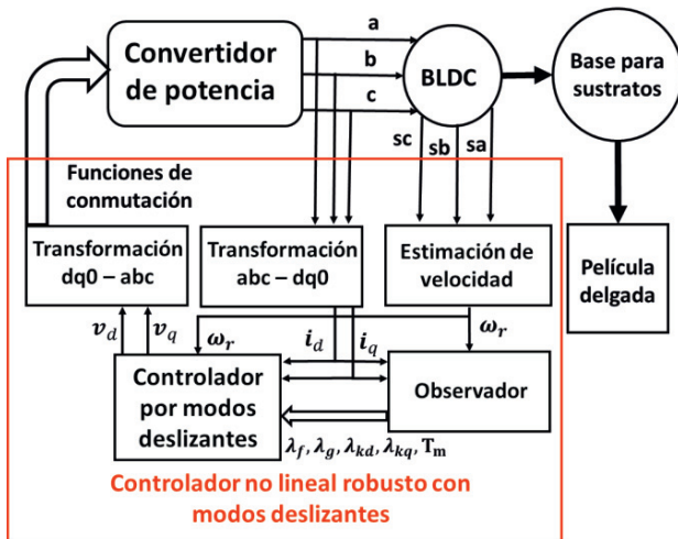
Figura 3: Diagrama a bloques del controlador por modos deslizantes propuesto.
