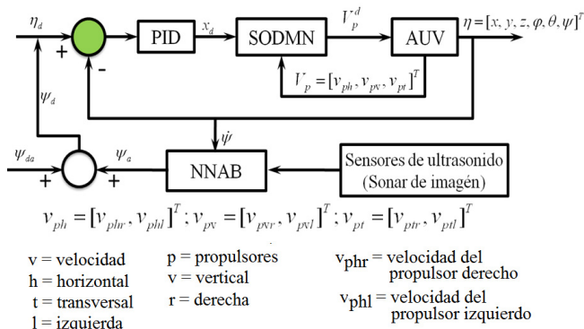
Figura 8. Esquema neuronal para el control de movimiento (SODMN) y la evasión de obstáculos reactiva (NNAB).
