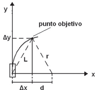
Figura 6: Ley de persecución pura. (Ollero, 2001).
