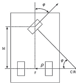
Figura 5: Esquema cinemática AGV.
