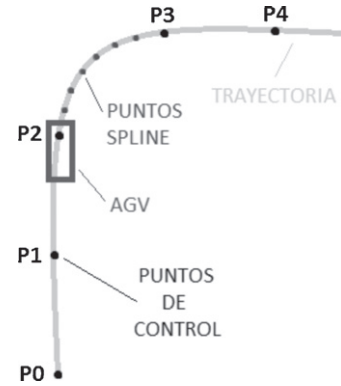
Figura 7: Ejemplo de definición de puntos de control de la trayectoria e interpolación mediante splines entre punto P2 y P3
