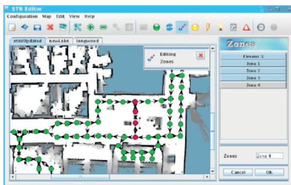
Figura 12: Editor en modo de edición de zonas.
