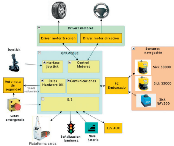
Figura 3: Arquitectura hardware de un AGV.
