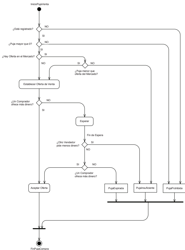
Figura 7: Diagrama de actividad del algoritmo de procesado de una puja de venta
