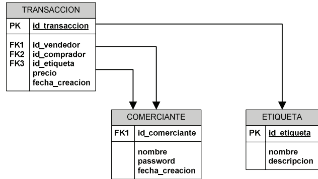
Figura 9: Modelo de información persistente: estructura de la base de datos
