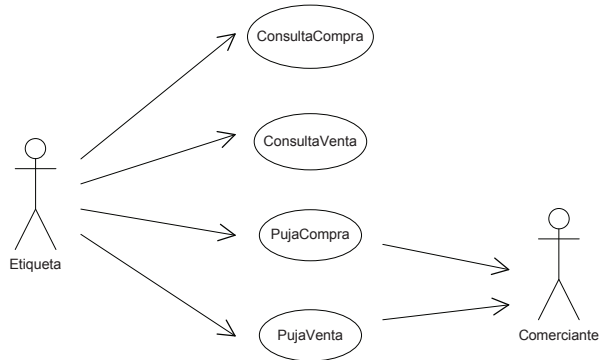
Figura 5: Casos de uso relacionados con el proceso de subasta
