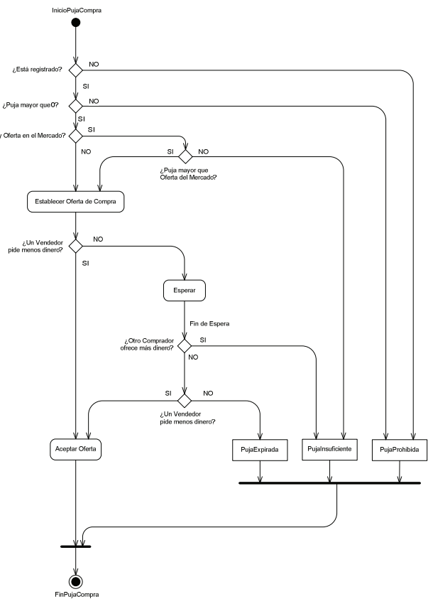
Figura 6: Algoritmo de procesamiento de una puja de compra
