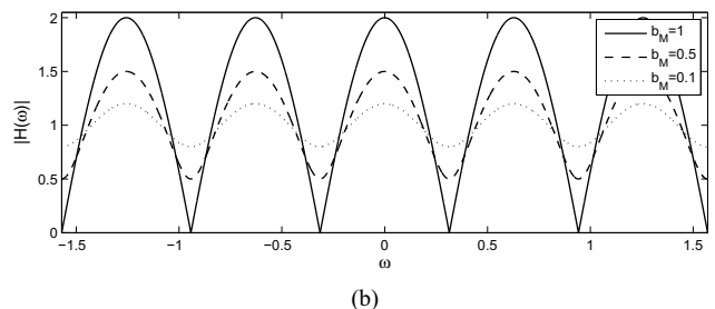
Figura 2. Filtro Feedforward Comb . (a) Esquema. (b) Respuesta en frecuencia.
