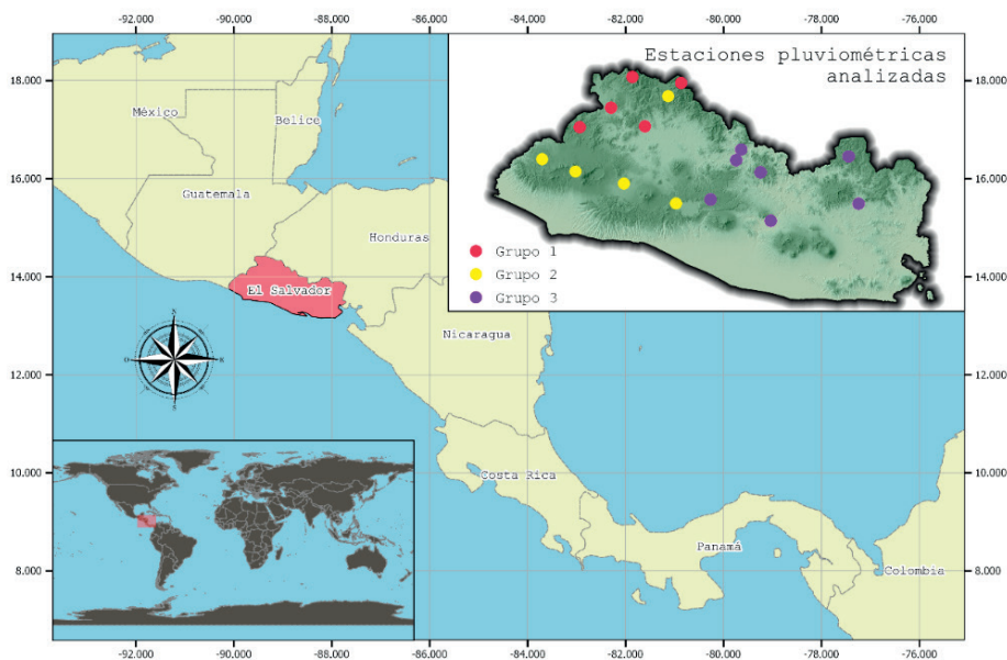
Figura 1. Ubicación de las estaciones meteorológicas en el mapa de relieve de El Salvador y su ubicación en Centro América y el mundo.
