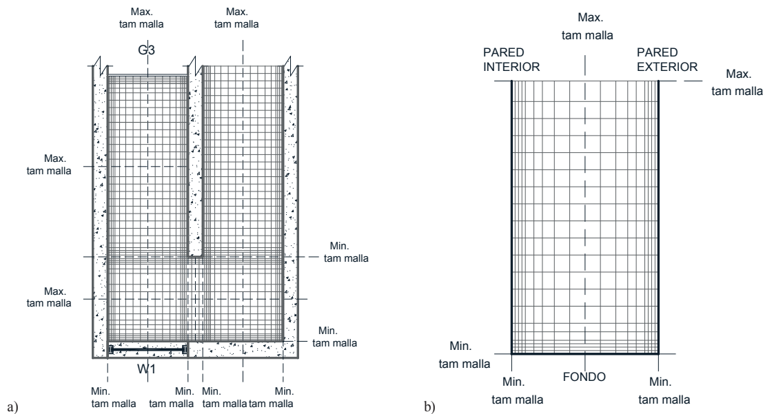
Figura 3 | Configuración del malla, a) vista en planta – detalle de la parte curva b) perfil de sección transversal.
