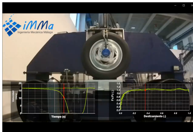
Figura 1: Banco de ensayo de neumáticos. Video del ensayo longitudinal con los datos superpuestos.
