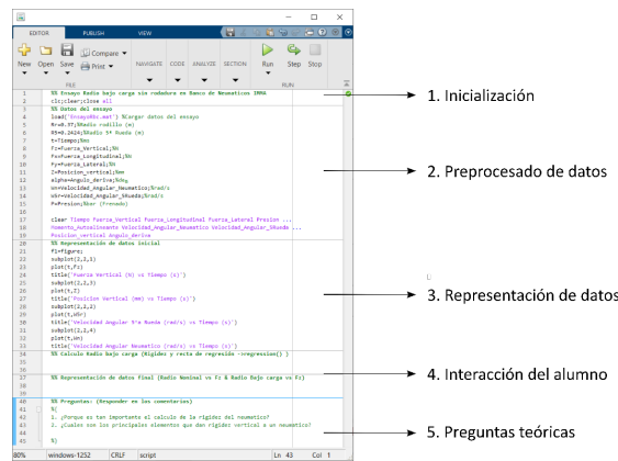
Figura 3: Plantilla MATLAB.
