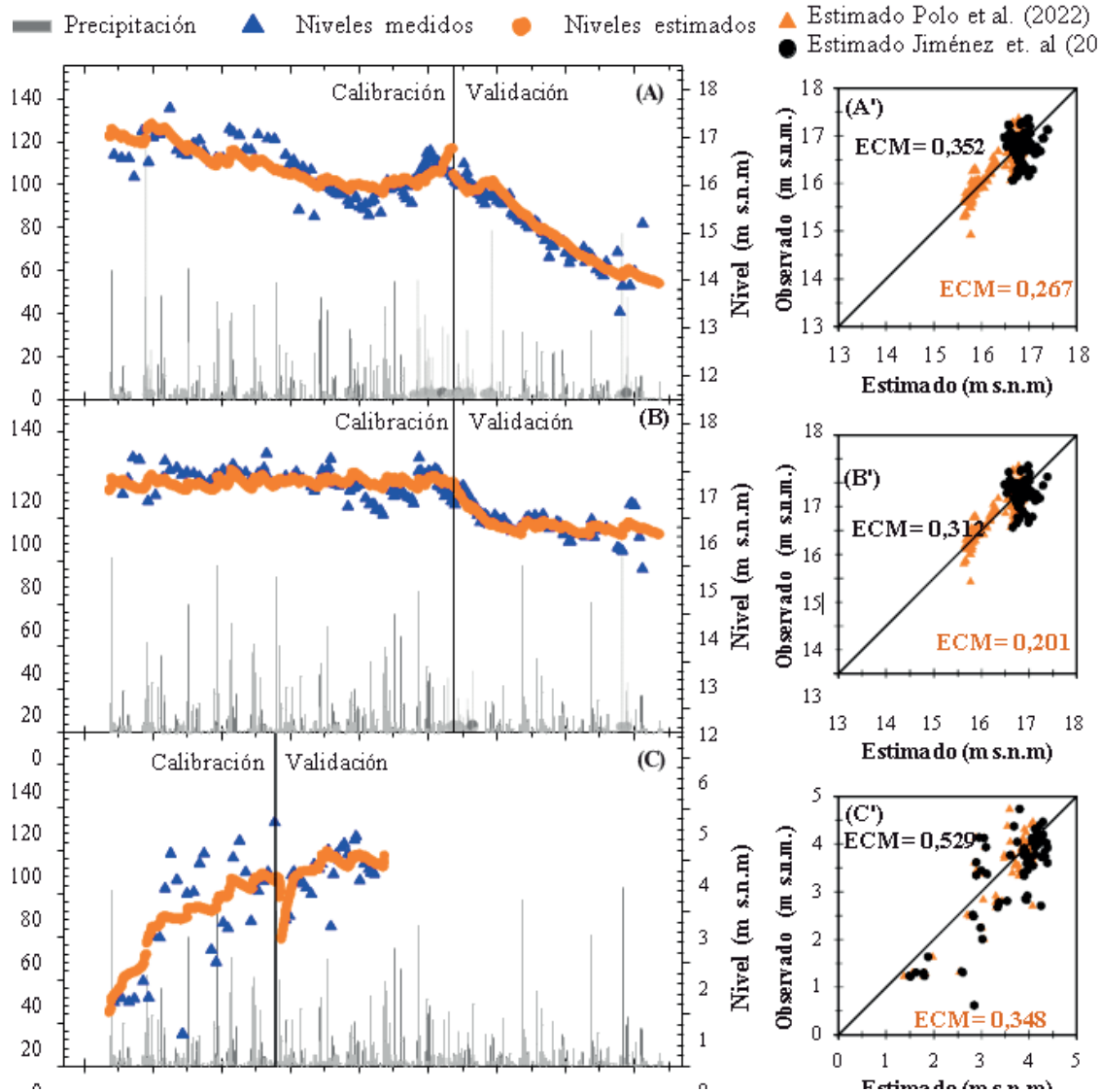
Figura 1 | Izquierda: Ajuste de niveles piezométricos durante los periodos de calibración y validación para áreas dedicadas al cultivo de cítricos (A), cultivos anuales (B) y cultivos perennes (C). Derecha: Relación entre los valores calculados y observados, comparando los resultados obtenidos por Jiménez-Martínez et al. (2010) (círculos negros) con los derivados de nuevos parámetros usados para cítricos (A'), cultivos anuales (B') y cultivos perennes (C') (triángulos anaranjados) por Polo (2022). CME: error cuadrático medio.
