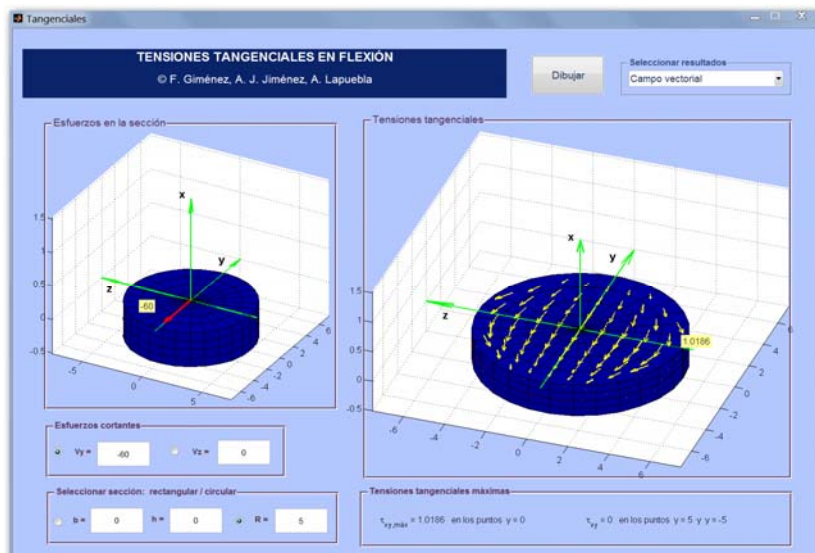
Fig. 5. Ejemplo de uso: sección circular, campo vectorial
