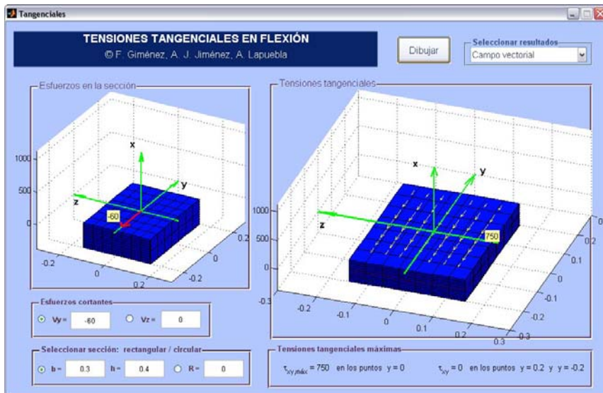
Fig. 3. Ejemplo de uso: sección rectangular, campo vectorial
