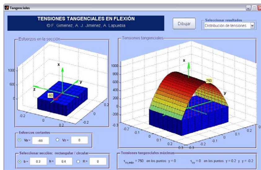
Fig. 2. Ejemplo de uso: sección rectangular, distribución de tensiones
