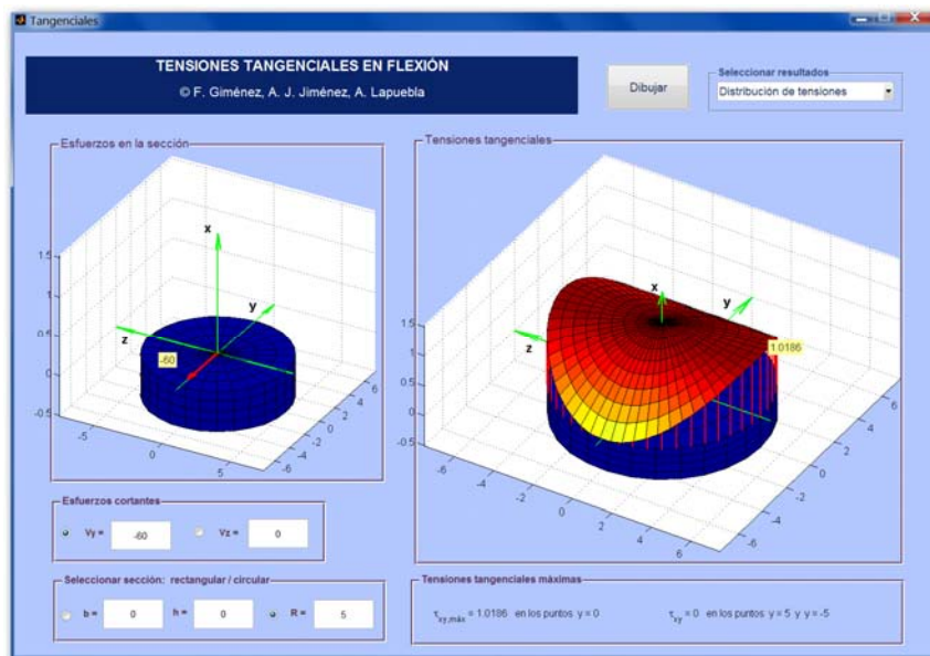
Fig. 4. Ejemplo de uso: sección circular, distribución de tensiones
