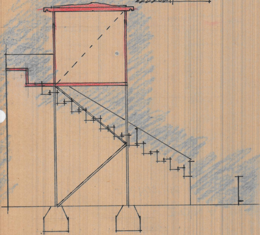
CABINA SECCION AB
